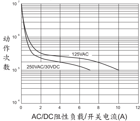
预期寿命
