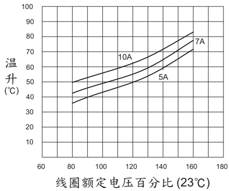
线圈温升
